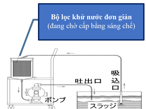
< Sơ đồ quy trình thiết bị >
