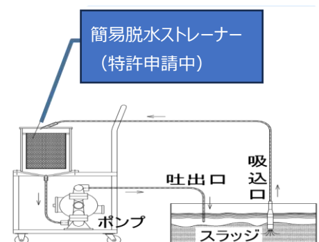
<装置フロー図>
